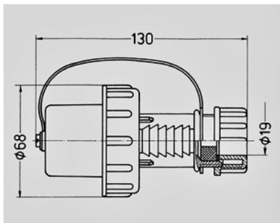
Zeichnung 2 MB 163
